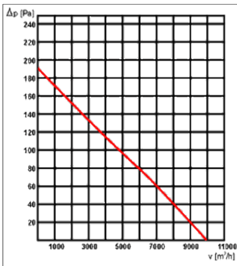
WOD-K-630
