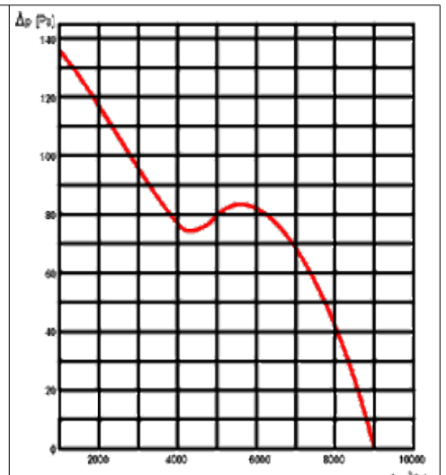
WOD-K-560
