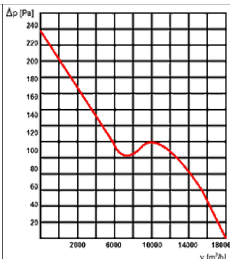
WOD-K-710
