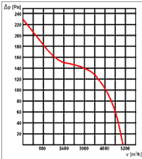
WOD-K-450
