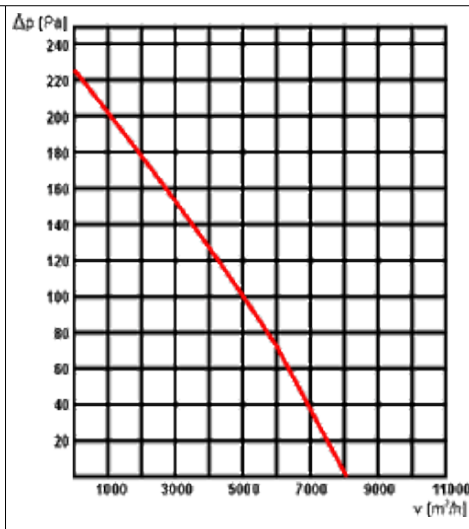
WOD-K-500
