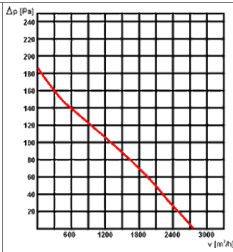
WOD-K-355
