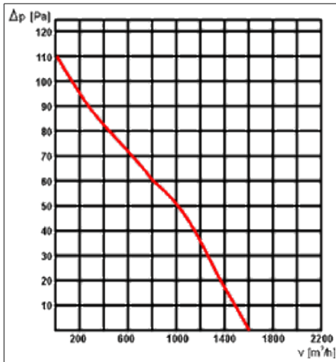
WOD-K-315
