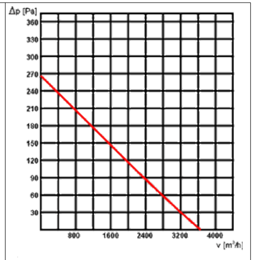
WOD-K-400
