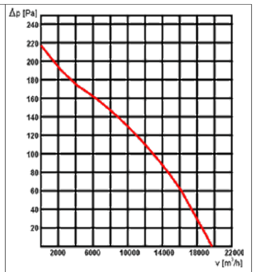
WOD-K-800
